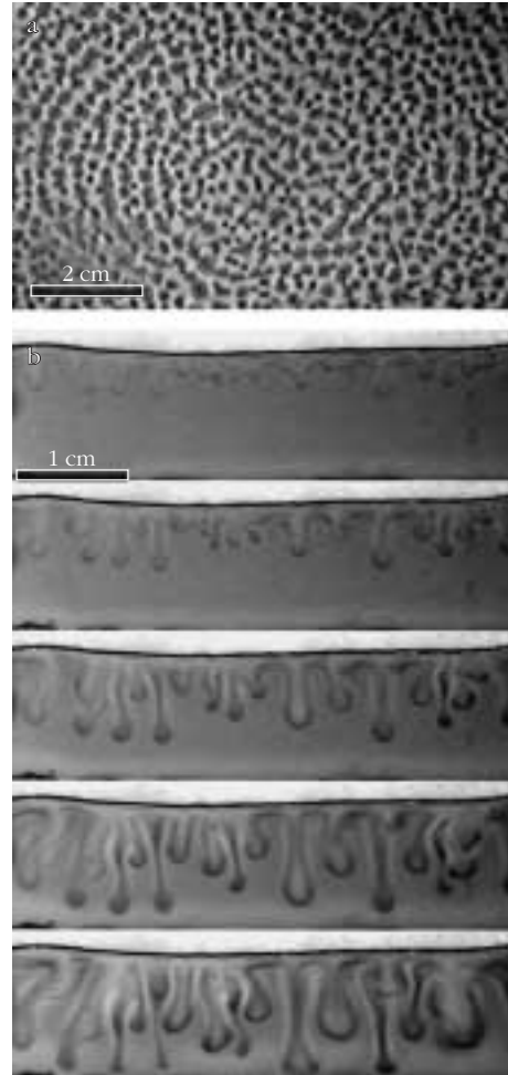
1. ábra. Biokonvekció Bacillus subtilis folyadék-kultúrákban. a: Petri-csészében kialakuló mintázat felülnézete. b: Hele-Shaw-cella oldalnézete és az instabilitás időfejlődése félperces időközönként. A sötétebb területeken nagyobb a baktériumok száma. [1] alapján.
