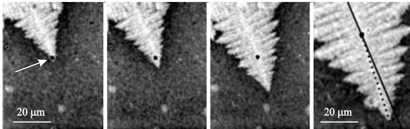
8. ábra. A dendritcsúcs szennyező szemcse által okozott eltérése a kísérletekben (J.F. Douglas és V. Ferreira szívességéből). Vegyük észre a dendrit gerincének és oldalágainak irányváltását, ami új orientáció megjelenésére utal.
