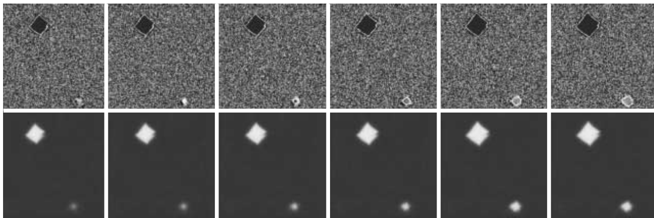
6. ábra. Zajindukált kristálynukleáció a fázismező-modellben a felületi szabadenergia négyfogatúsú szimmetriája mellett. Felső sor: orientációs térkép; alsó sor: fázismező-térkép.
