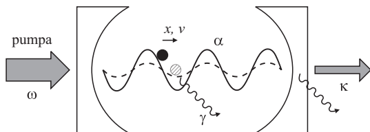
7. ábra. A mozgó atom megváltoztatja a rezonátorban kialakuló teret (intenzitását és fázisát), ami az atomi hely- és sebességváltozók ( x , v ) és a tér amplitúdója ( \alpha ) között bonyolult dinamikát hoz létre.
